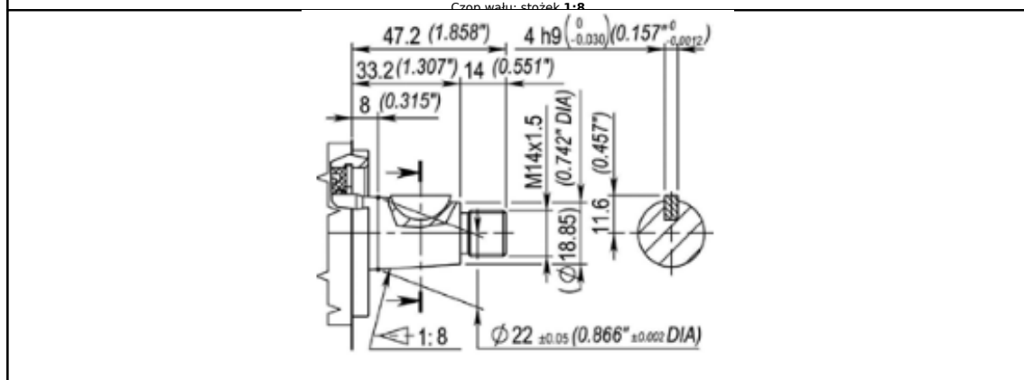
Czop walu: czołek 1:8
