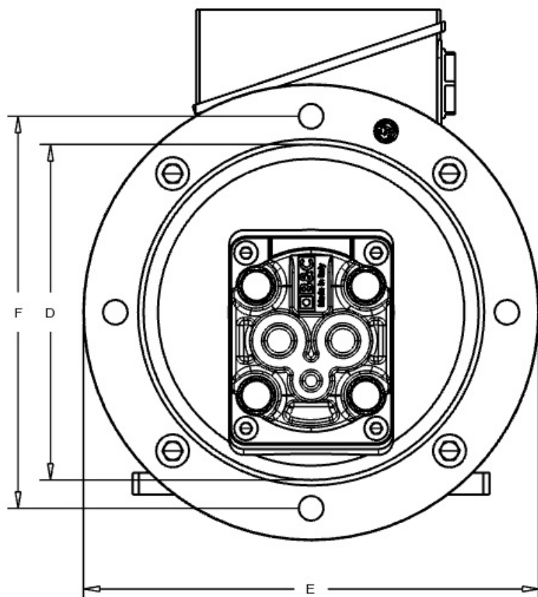
Zestawienie wymiarów zespołów pompowych zębatych
