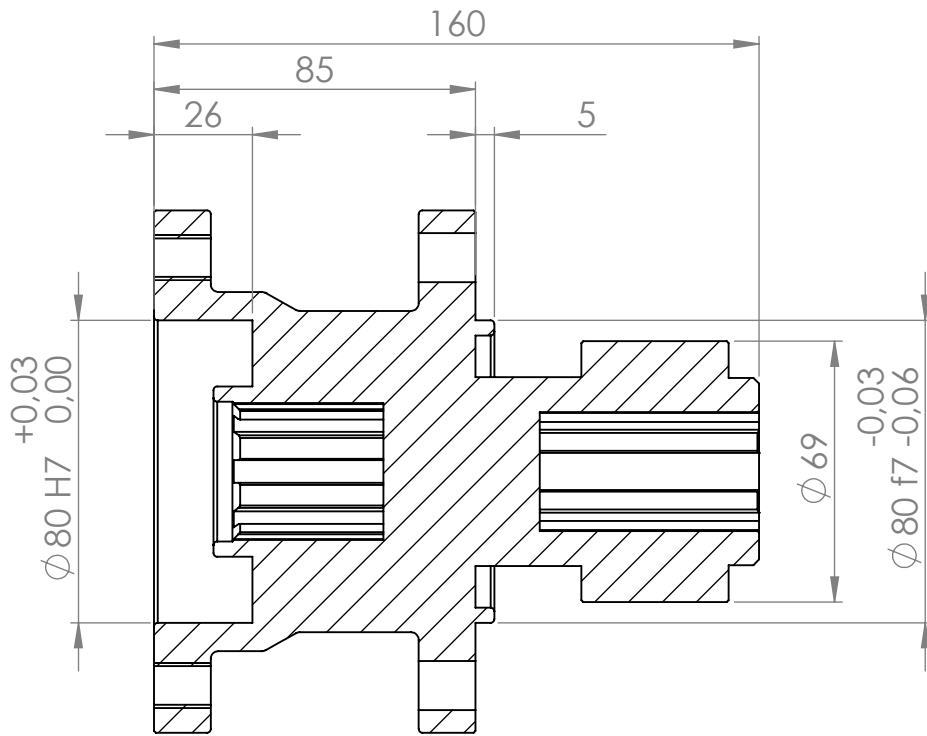
PRZEKRÓJ A-A SKALA 1 : 2
