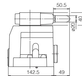
AGIS-32; Mass = 9,9 Kg AGIU-32; Mass = 9,9 Kg
