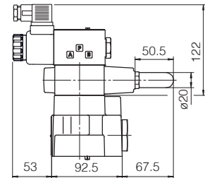
AGIU-10/**-LX Mass = 5,4 Kg
