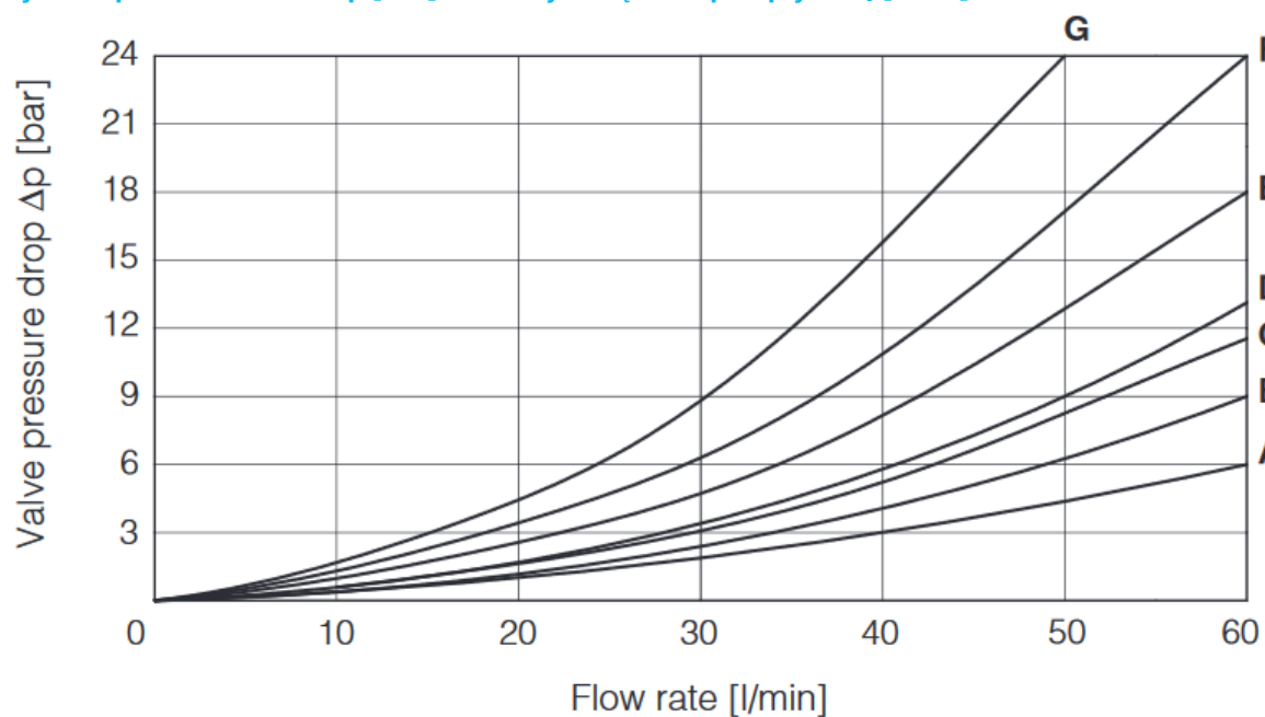
Wykres spadku ciśnienia \Delta p [bar] w funkcji natężenia przepływu Q [l/min]
