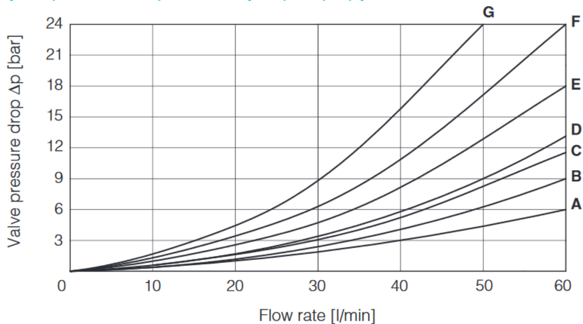
Wykres spadku ciśnienia \Delta p [bar] w funkcji natężenia przepływu Q [l/min]
