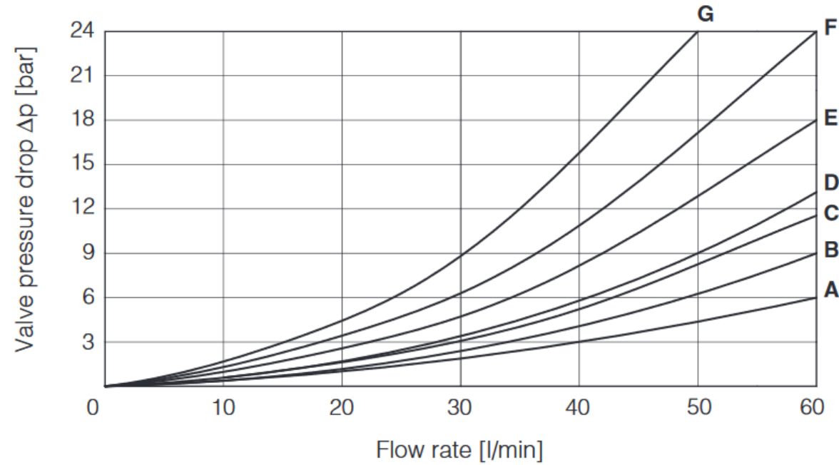
Wykres spadku ciśnienia Δp [bar] w funkcji natężenia przepływu Q [l/min]
